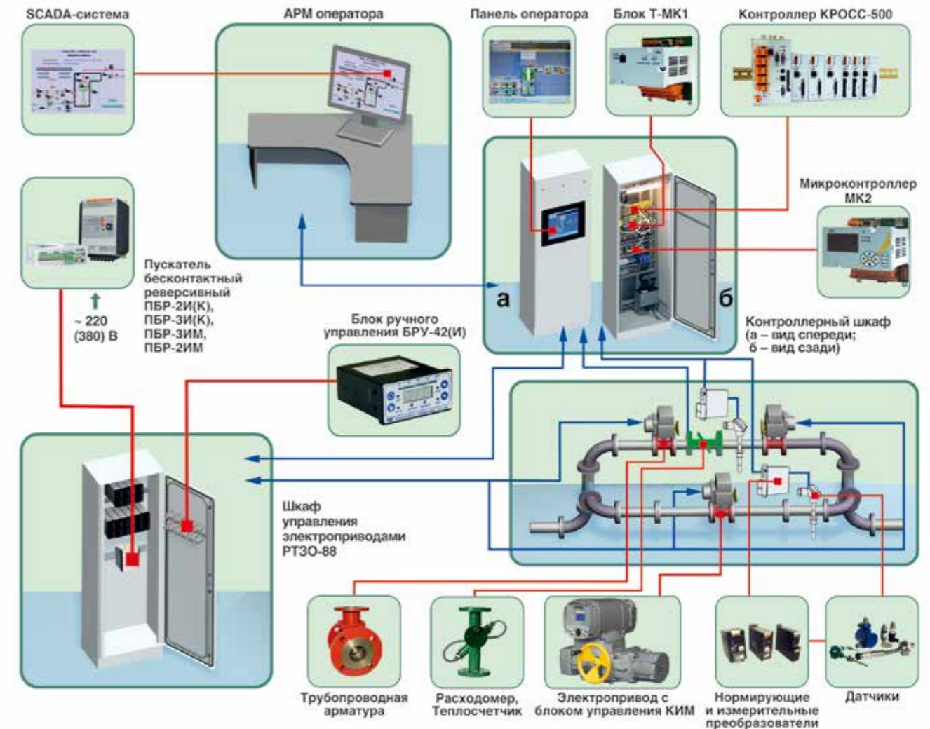
Рис. 1 Система диспетчерского управления на базе оборудования «АБС ЗЭИМ Автоматизация»
